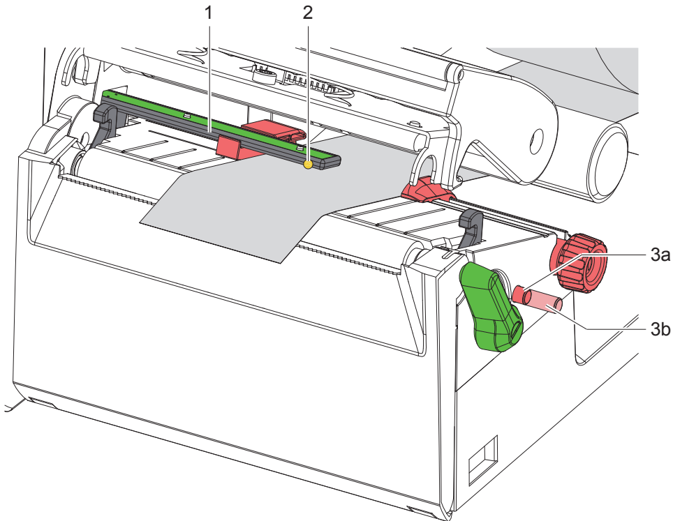
Bild 10 Etikettenlichtschanke einstellen
