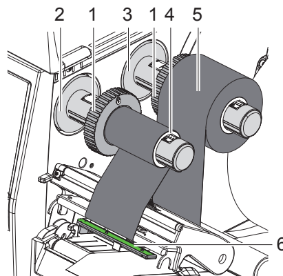
Bild 12 Transferfolie einlegen
