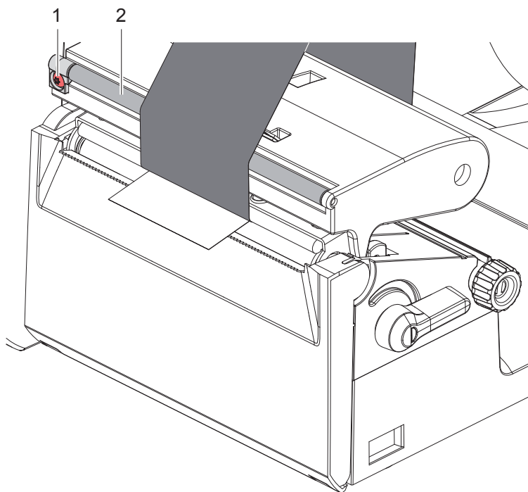
Bild 14 Transferfolienlauf einstellen
