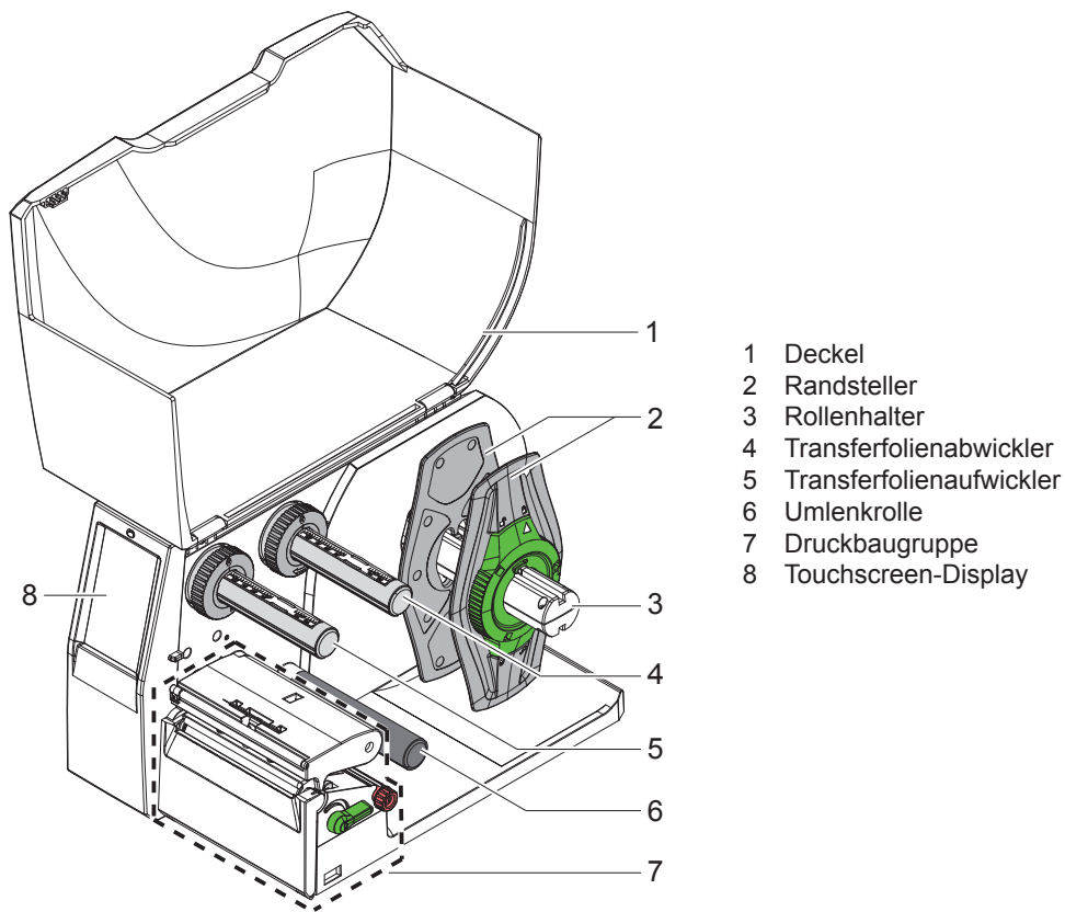
Bild 1 Übersicht
