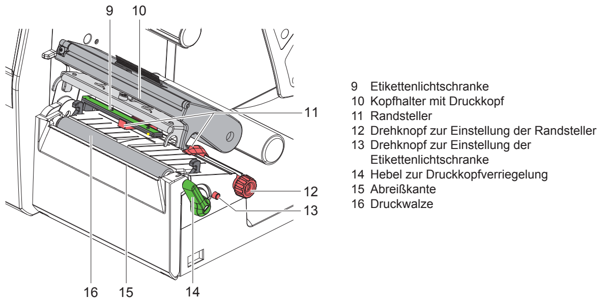
Bild 2 Druckbaugruppe
